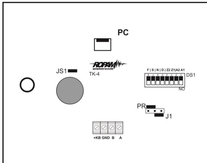
2. Widok płytki PCB.
